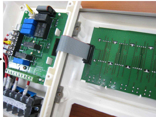
9. 본체에 나와있는 연결 케이블을 방향에 맞추어 전면케이스와 결합합니다.
