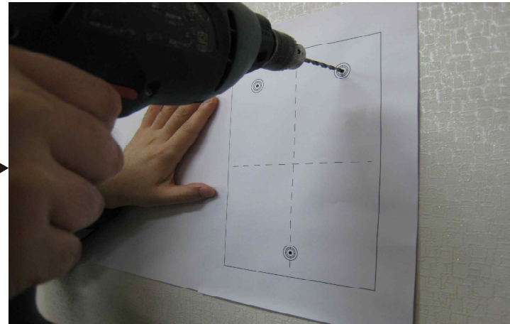
5. 설명서 뒷편의 타공홀 가이드를 이용하여 설치할 철판에 미리 홀을 뚫습니다.
