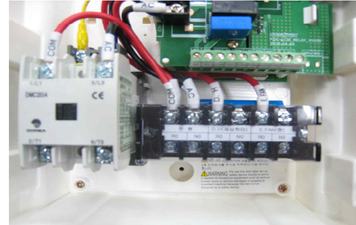
2. 동봉된 설명서나 덮개 뒷편의 단자 스티커를 참고하여 배선작업할 부분을 확인합니다.
