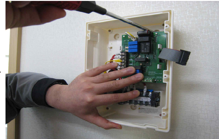
6. 5번에서 뚫어놓은 홀에 맞추어 제품을 부착합니다. (4*20mm 피스)
