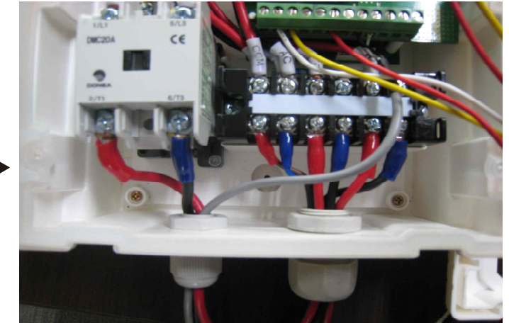
7. 각종 장비를 연결하고 선작업을 마칩니다.
